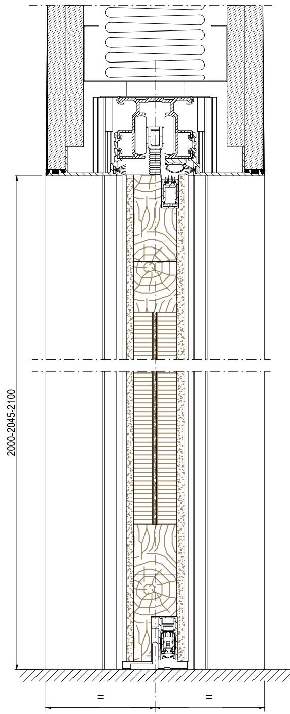
Sezione B-B (150 2L) Section B-B (150 2 D) Section B-B (150 2L)
