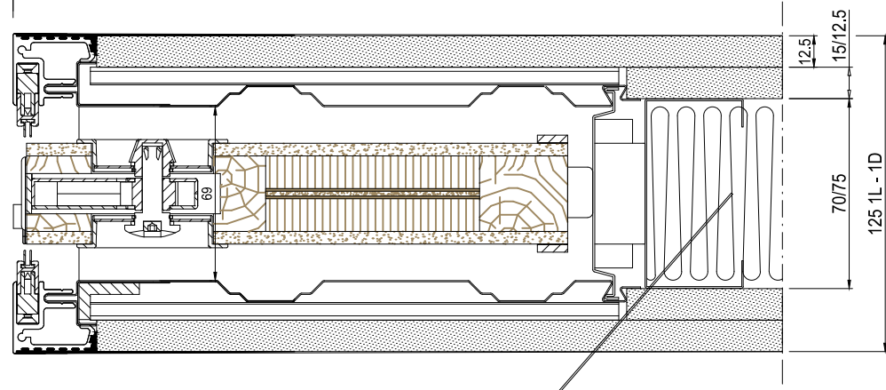
Sezione orizzontale 125 1L porta aperta Section horizontale 125 1 D porte ouverte Horizontal section one 125 Panel open door
