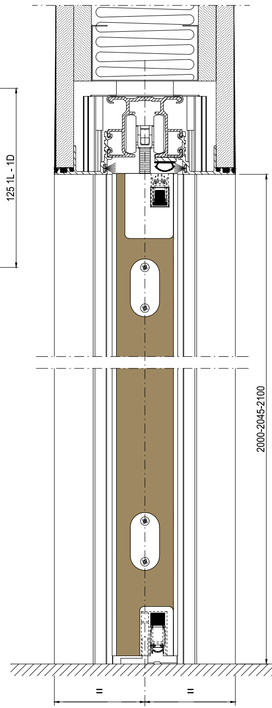
Sezione A-A (125 1L) Section A-A (125 1 D) Section A-A (125 1L)
