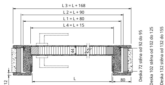
Deska 102 Tloušťka stěny min. 102 max. 125
