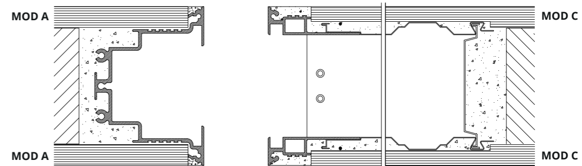
MONTÁŽ S POSUVNÝM ESSENTIAL / TECHZERO / MAGNIFICO FIT / 125 OMÍTKA
