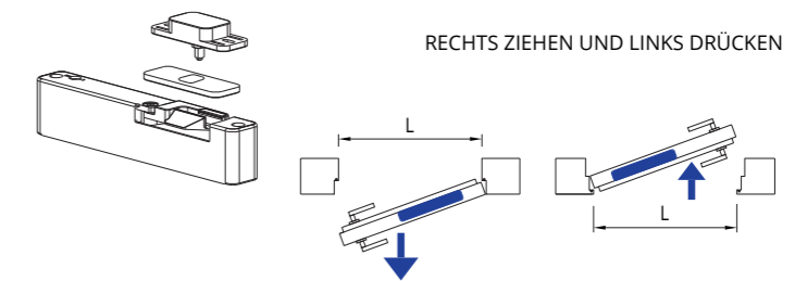
51297 Soft-Close TDX-SSX (270-017-563)
