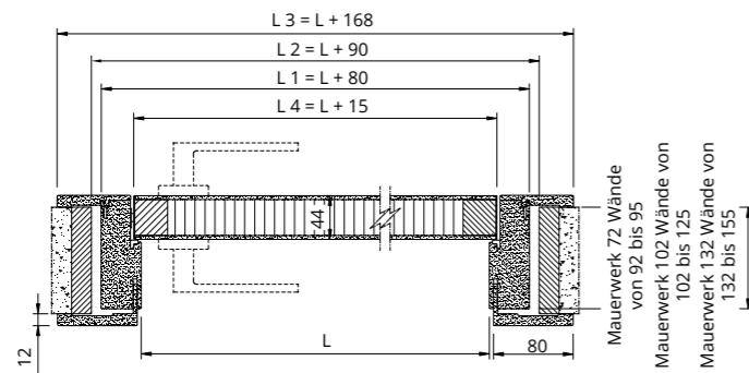
Mauerwerk 102 Wandstärke min. 102 max. 125
