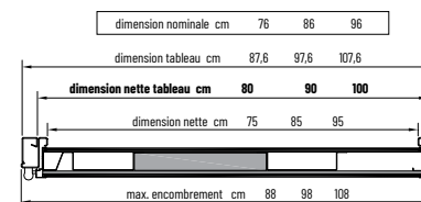
SECTION HORIZONTALE
